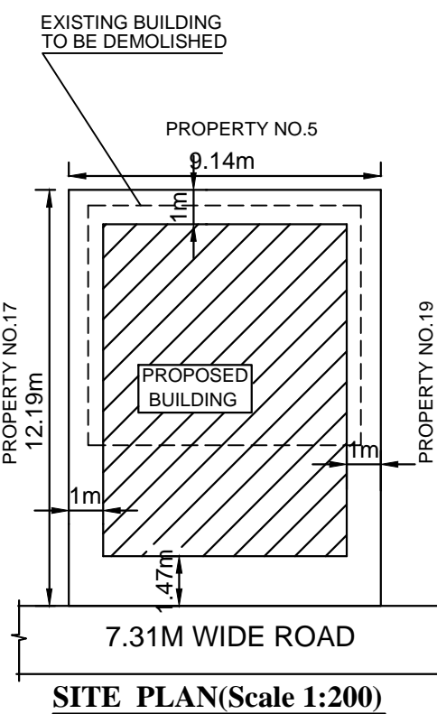
SITE PLAN(Scale 1:200)
